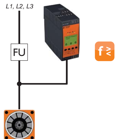
Sichere sensorlose Antriebsüberwachung durch Überwachung der Ausgangsfrequenz des Umrichters
